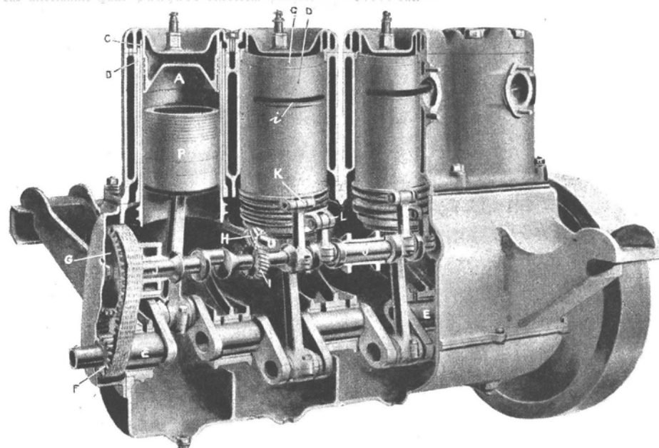
Schnitt des Schieberventilmotors Panhard-Knight. Der von Panhard & Levassor gebaute Schieberventilmotor. Details über die Arbeitsweise der Schieberbüfien. A Zylinderboden, CD Schieberbüfien, i Schlit, P Kolben, E Kurvelwelle, F, G Verteilerkettenräder, HI Schraubenträder für den Magnet- und Pumpenantrieb, J Verteilerwelle, KL Gegenterlängen zur Besorgung der Schieberbüfien.
